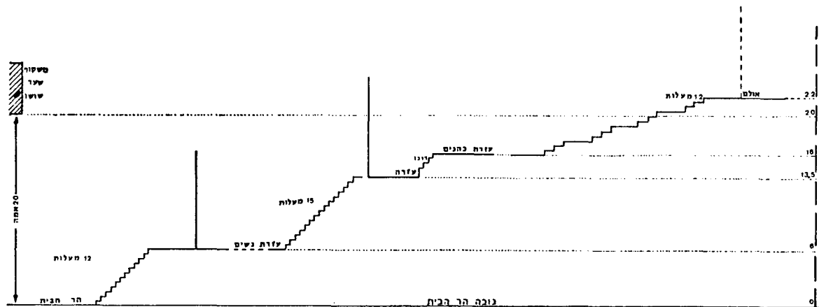
תמונה 15: תרשים הגבהים של חלקי המקדש השונים על פי המשניות
