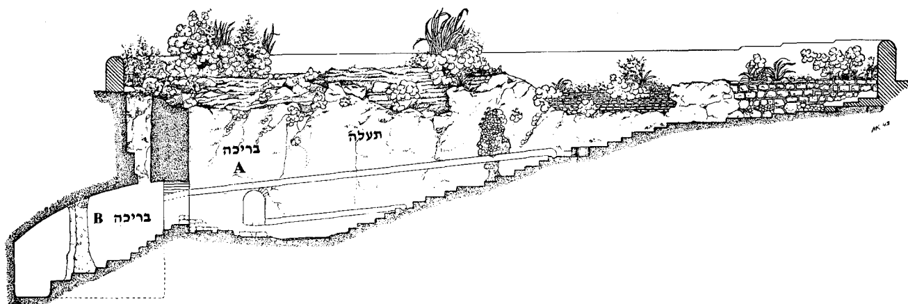
קברי מלכים חתך דרך מערכת המדרגות ומבט לתעלות החצובות בסלע והפתח לבריכה A
