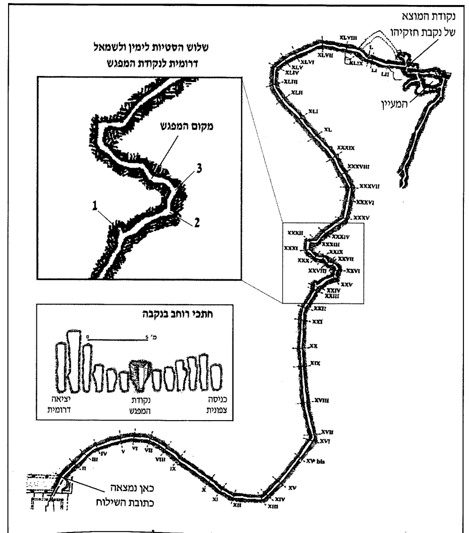
איור מספר 2: תוכנית ופרופיל של נקבת חזקיהו (על פי חלוקתו של ונסאן)
